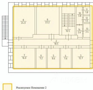
2-й этаж
