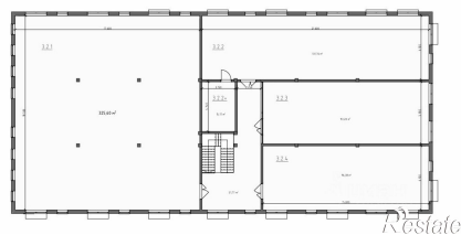
План 2 этажа
